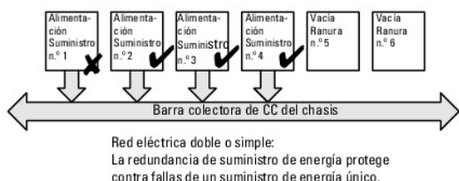
Figura 9-2. Redundancia de suministro de energía: total de 4 unidades de suministro de energía con la falla de una unidad.
