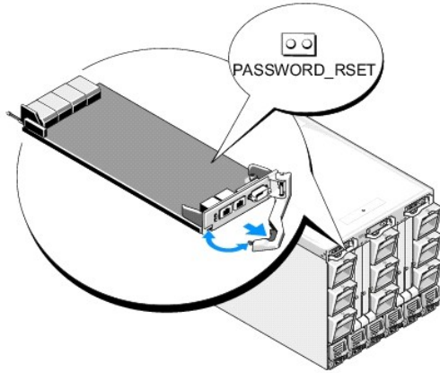
Figura 12-1. Ubicación del puente de restablecimiento de contraseña
