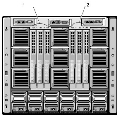
Figura 11-1. Vista posterior de un chasis, que muestra la ubicación de los módulos de E/S
