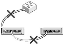
Figura 2-4. Cableado incorrecto para la conexión de red de CMC: Dos CMC
