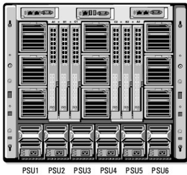
Figura 9-4. Configuración de chasis con seis unidades de suministro de energía
