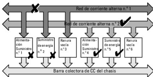
Figura 9-1. Figura 8-2. Dos unidades de suministro de energía por cada red eléctrica y una falla de alimentación en la red eléctrica 1
