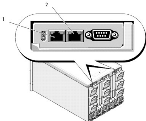
Figura 1-1. Chasis y CMC Dell M1000e
