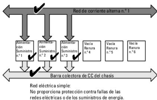
Figura 9-3. Sin redundancia con tres unidades de suministro de energía en el chasis
